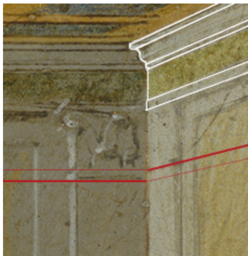
Fig. 46 Particolare delle linee d'imposta dei capitelli sfalsate (in rosso) e l'ipotesi formulata sulle modanature della cornice soprastante (in bianco).
