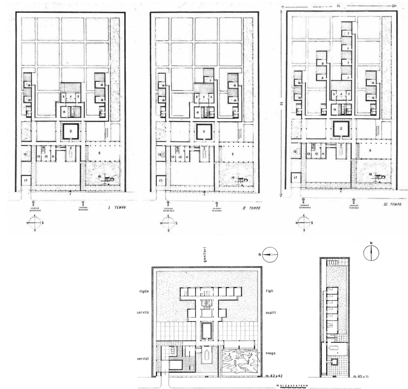
Arch. Cesare Cattaneo - Pianta della Casa-Famiglia media e popolare.
