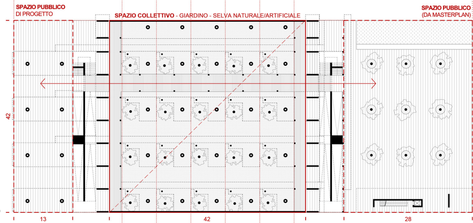
PROGETTO - pianta +/-0,00
