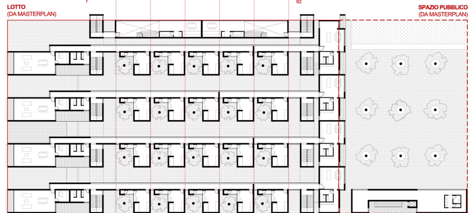
PROGETTO - pianta +7,50
