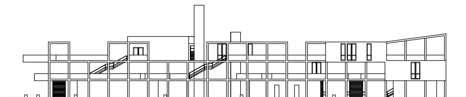
SEZIONE BB'
