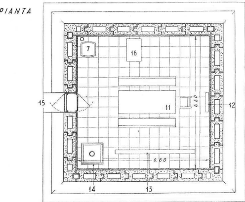
Arch. Cesare Cattaneo - Sala della Famiglia. Sezione e pianta.
